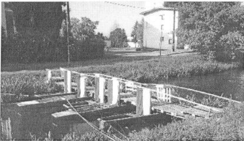
Lávka přes rameno řeky Moravy na Vodním království 2016, stavba Vodní skauti Hodonín, hlavní projektant Michal „Pytlík“ Kordík
